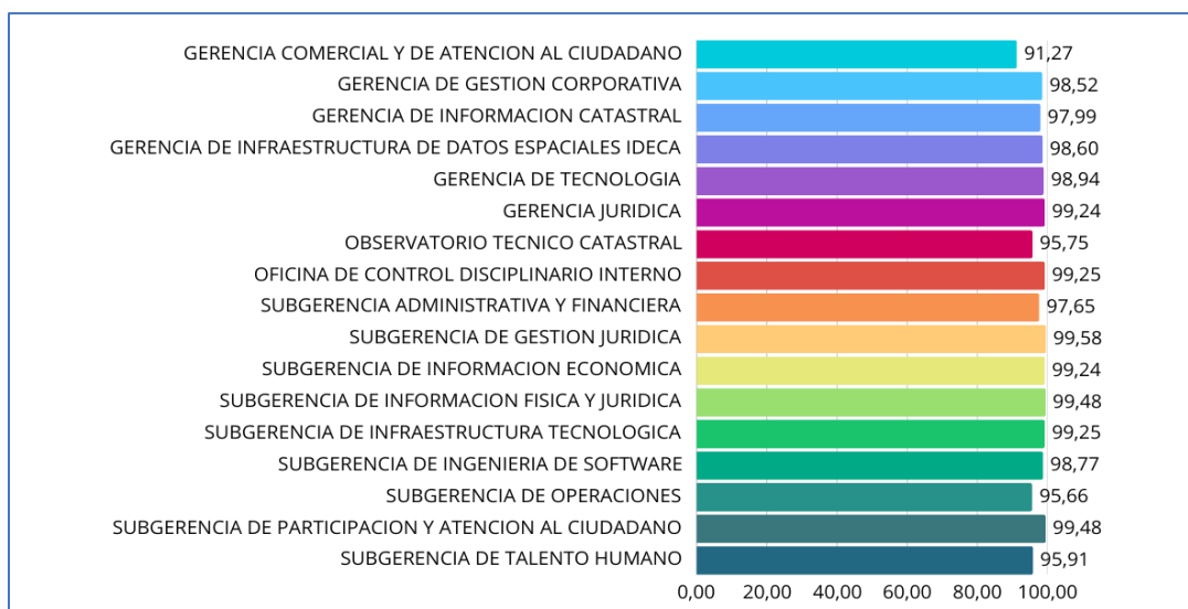
Gráfica 4: Resultados calificación acuerdos de gestión 2024 – UAEC
